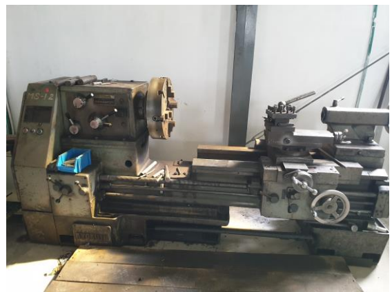
Máy tiện - KYOKUTO Chiều dài chống tâm: 1300 mm Đường kính tiện qua băng: 600 mm
